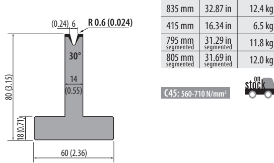
T80.06.30 350 kN/m max.
