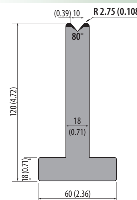
T120.10.80 950 kN/m max.
