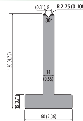
T120.08.80 950 kN/m max.
