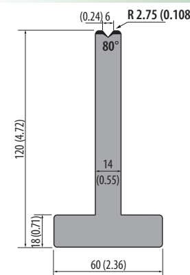
T120.06.80 950 kN/m max.
