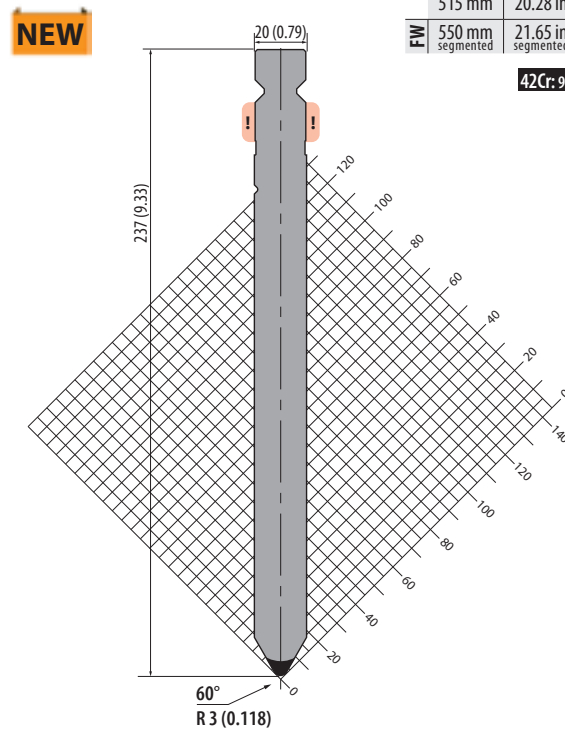
TPR237.60.R3
