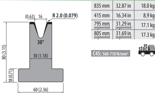
T80.16.30 450 kN/m max.
