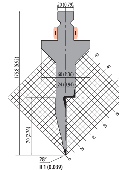
TPR176.28.R1
