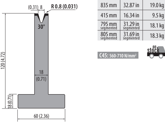
T120.12.30 400 kN/m max.
