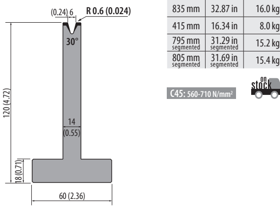
T120.10.30 500 kN/m max.
