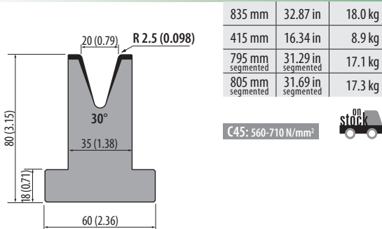
T80.20.30 500 kN/m max.
