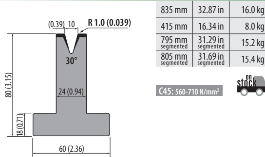
T80.10.30 500 kN/m max.
