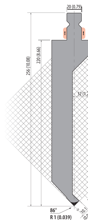
TPR256.86.R1-A
