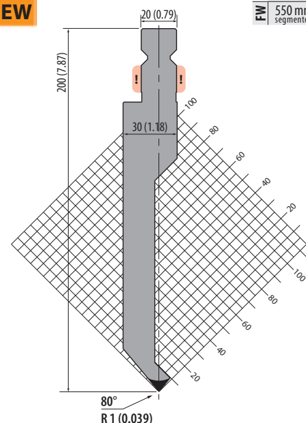
TPR200.80.R1
