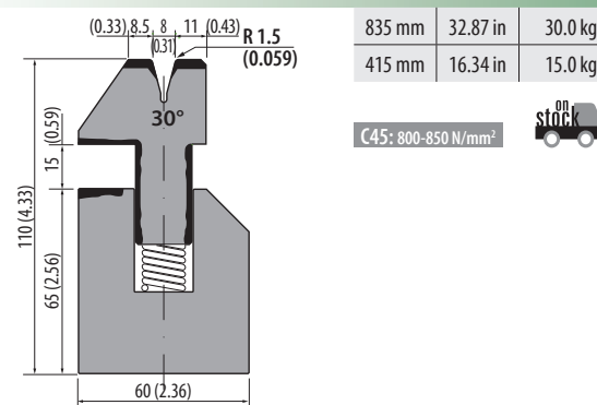
S110.30.08 800 kN/m max.
