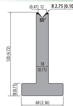
T120.12.80 950 kN/m max.
