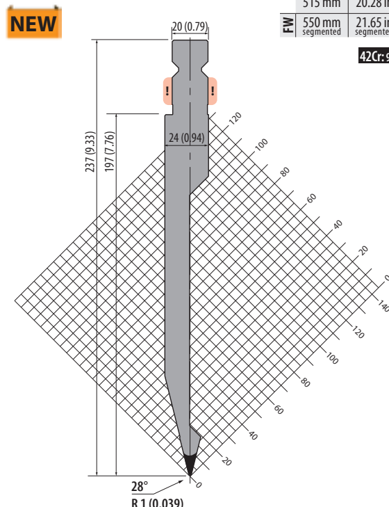
TPR237.28.R1
