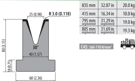
T80.25.30 500 kN/m max.
