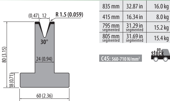
T80.12.30 400 kN/m max.
