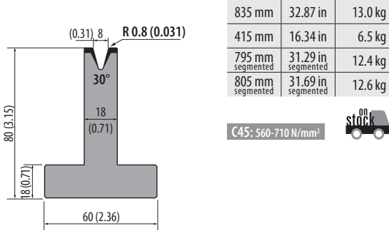
T80.08.30 350 kN/m max.
